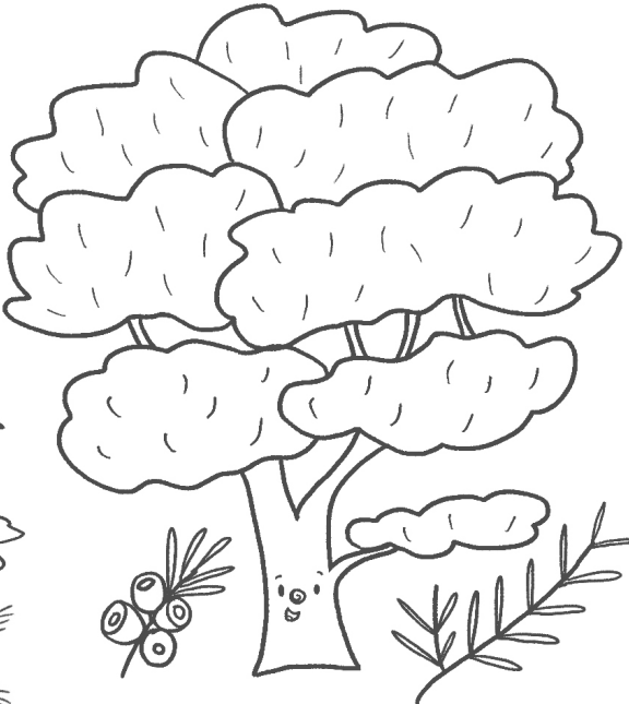
Yew
