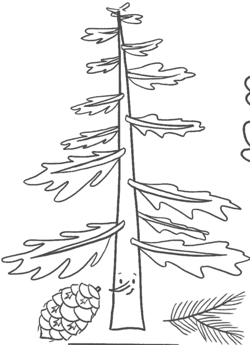
Douglas Fir
